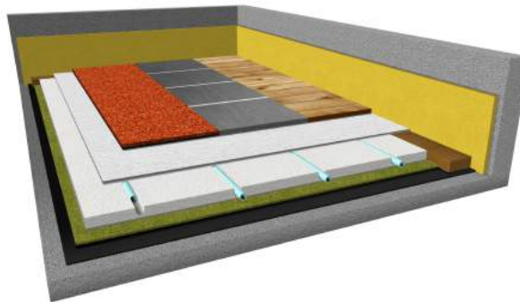
Płyta systemowa gipsowo-włókninowa - element prosty Gypsum-fiber board - straight element
