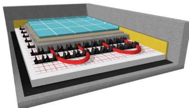
Szyny do montażu rur ogrzewania podłogowego Mounting rails for underfloor heating pipes
