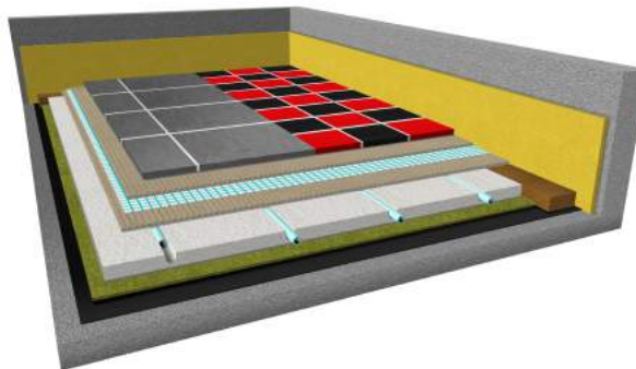
Płyta systemowa gipsowo - włókninowa - element skrętny Gypsum-fiber board - element with round pattern
