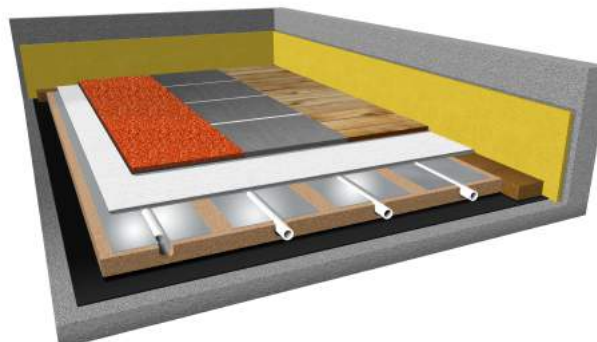
Płyta Acoustic - element skrętny Wood Fiber Board - element with round pattern
