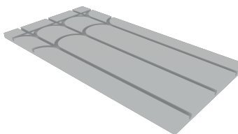
Płyta Sander Standard EPS - element prosty z podwójnym łukiem Sander Standard EPS board - straight element with double torsion ending
